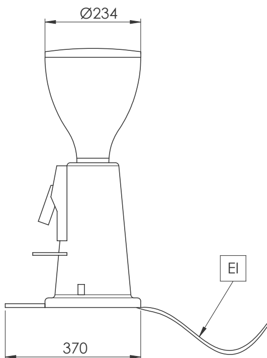
Zij aanzicht
